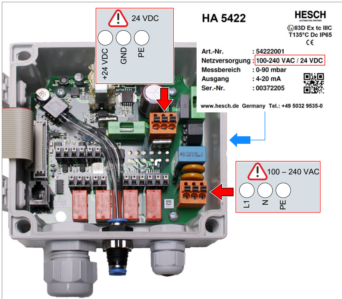
Abb. 5.1: Versorgungsspannung
