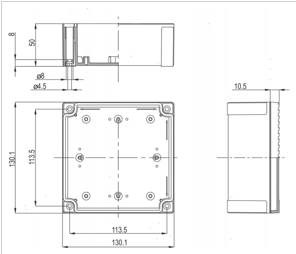
Abb. 4.1: Abmessungen
