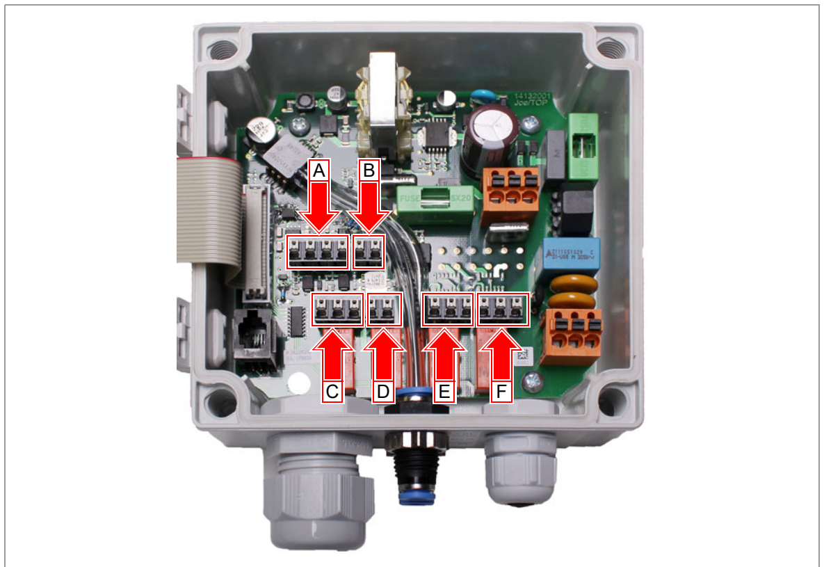
Abb. 7.1: Anschlussraum
