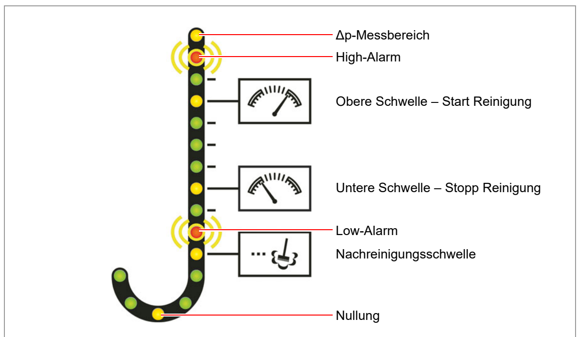
Abb. 3.3: Differenzdrucksäule
