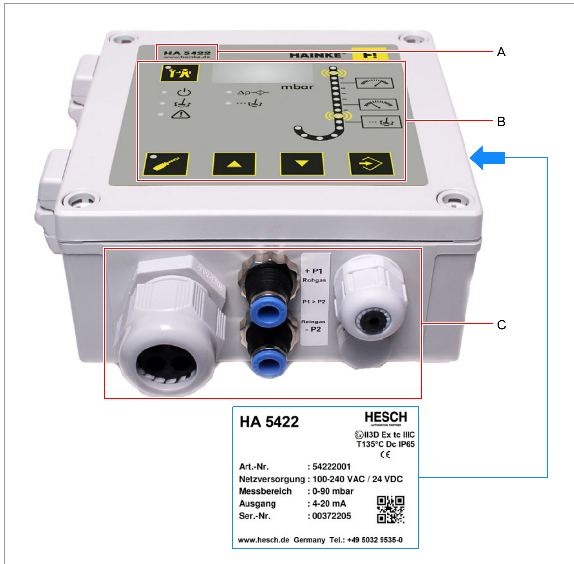
Abb. 3.1: Übersicht
